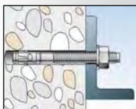
svorníková kotva FBN II
