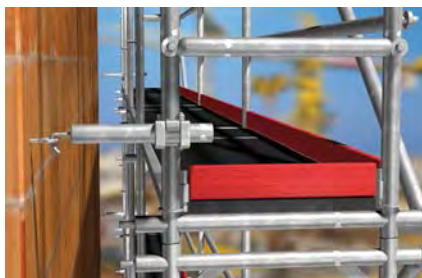
Fasádnická lešení
