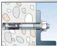
svorníková kotva FAZ II
