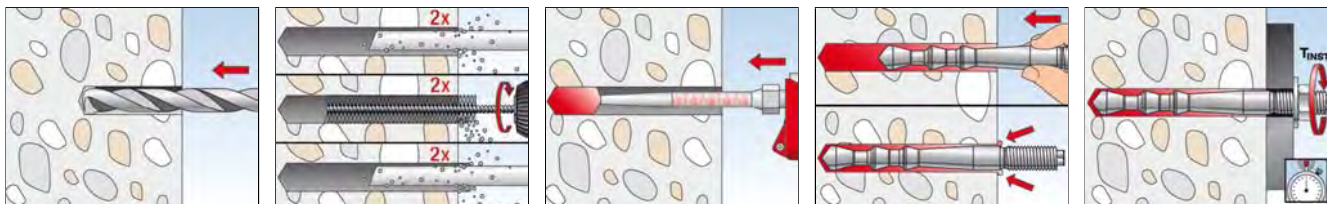
Chemická patrona FHB II-P (standardní)
