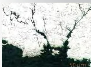
Příklad trhliny způsobené transkrystalickou korozi napětím v plechu 1.4401, který byl vystaven značně velkým účinkům chlórů..
