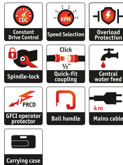
LW 1202 N 1600 W leštička za mokra na kámen se zástrčkou pro dělicí trafo, 130 mm Obj. č. 477.761
